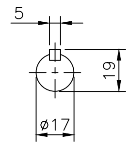
出力軸 Output Shaft
