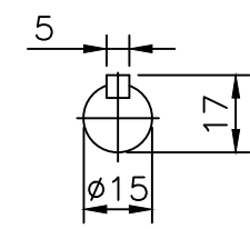
入力軸 Input Shaft
