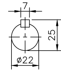
出力軸 Output Shaft
