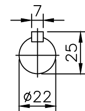
出力軸 Output Shaft
